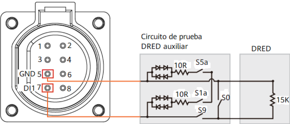
Figura 7-17 Diagrama de cableado de la función DRM
