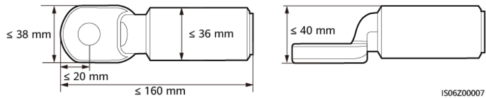
Figura 5-8 Especificaciones del terminal OT/DT engastado
