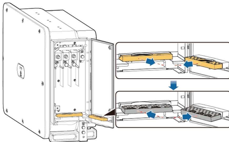
Figura 5-6 Reemplazo del módulo de crimpado
