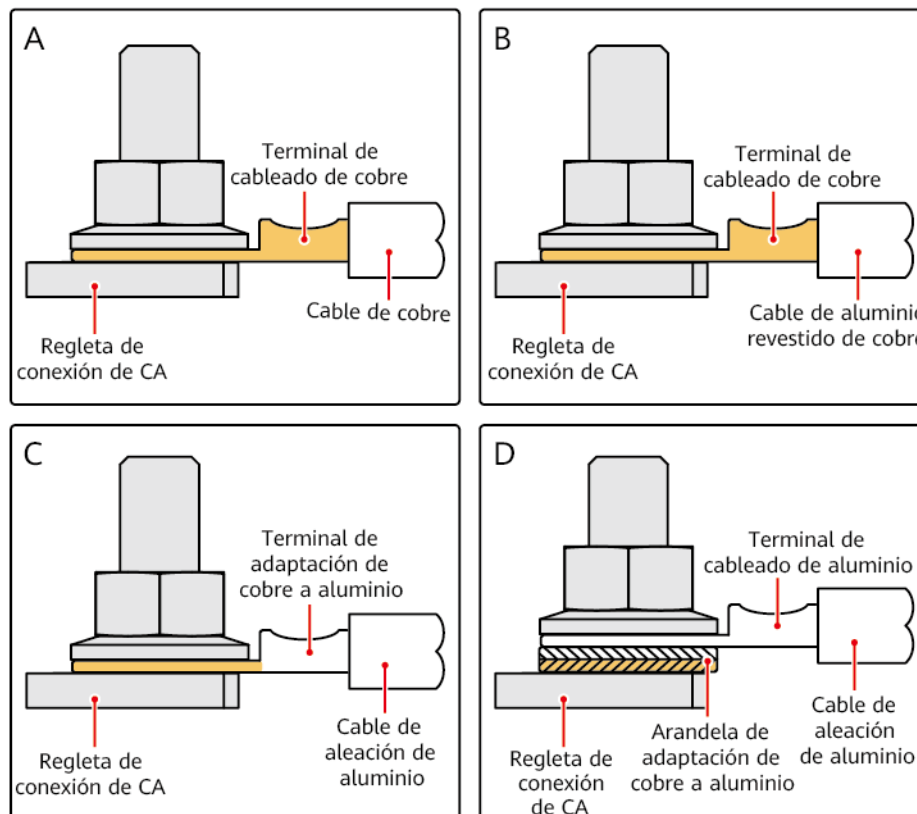
Figura 5-1 Requisitos para los terminales OT/DT
