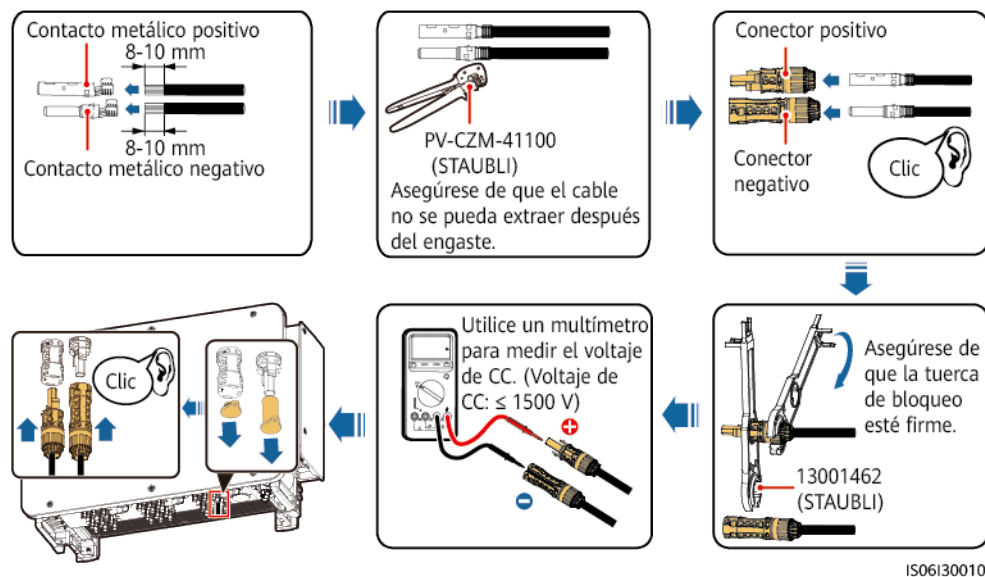
Figura 5-16 Conexión de cables
