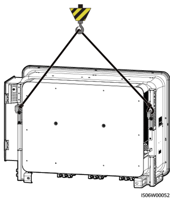
Figura 4-14 Elevación del inversor
