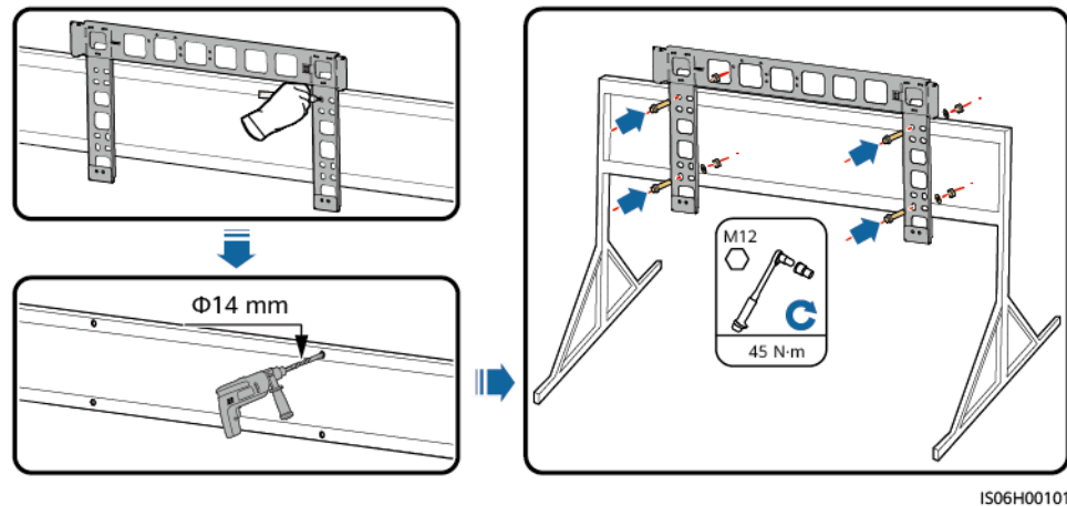
Figura 4-9 Cómo instalar la estructura de montaje
