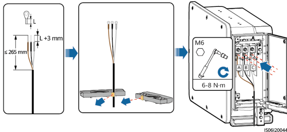
Figura 5-7 Conexión de cables
