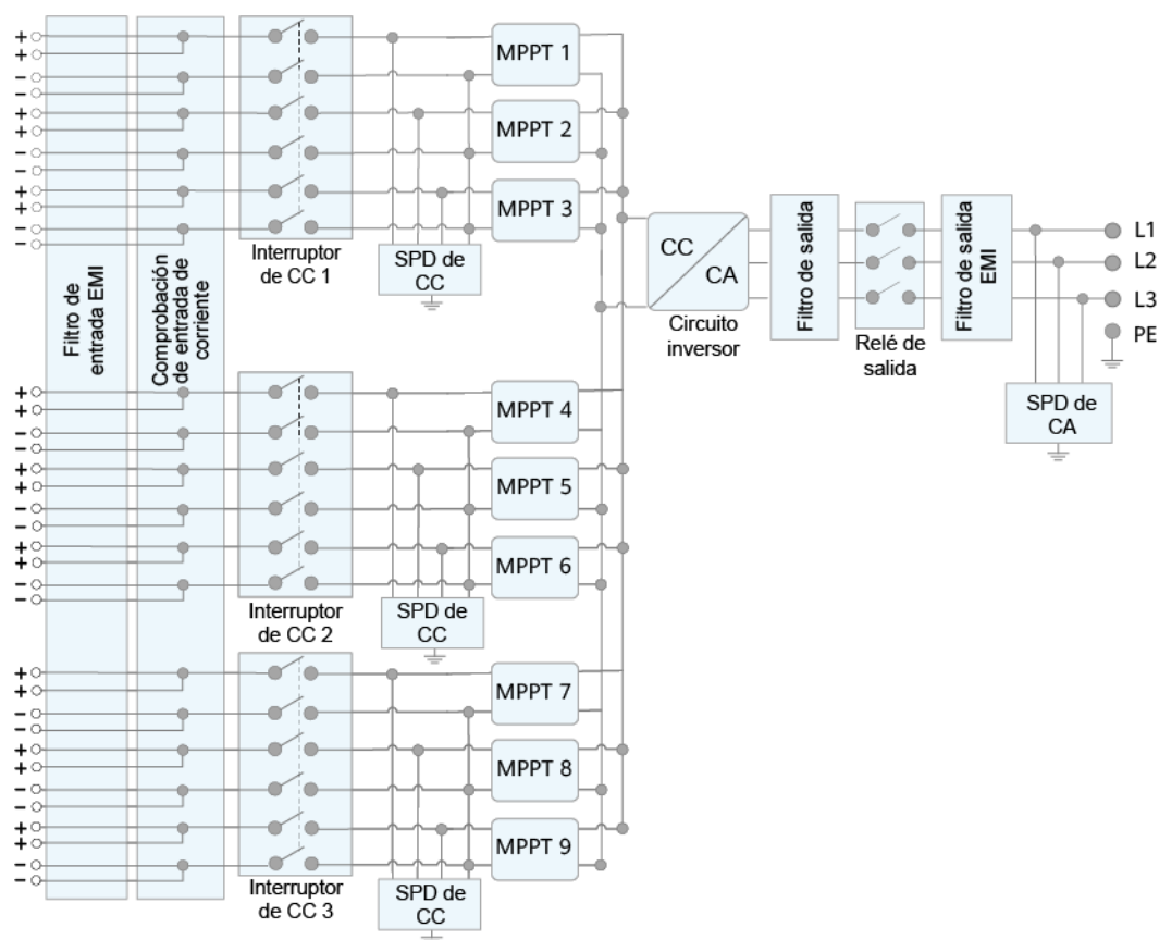
Figura 2-8 Diagrama conceptual del inversor
