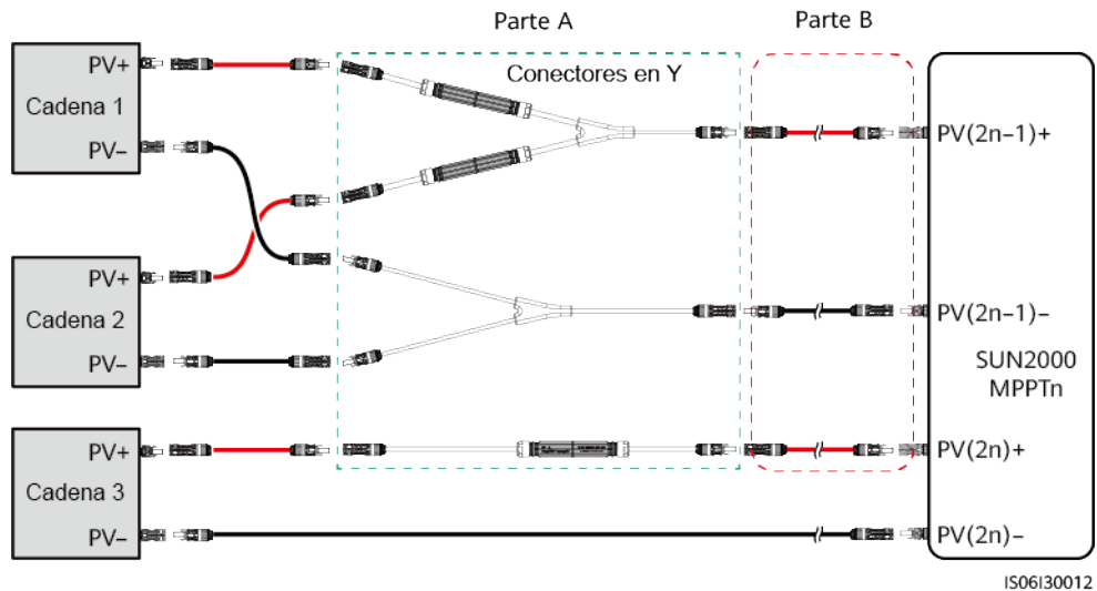
Figura 5-15 Solución de conectores de derivación en Y
