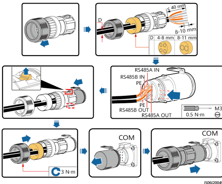
Figura 5-20 Conexión de cables (boquilla de goma de cuatro orificios de 4 a 8 mm)
