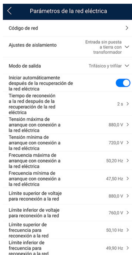
Figura 7-10 Parámetros de la red eléctrica (usuario especial)
