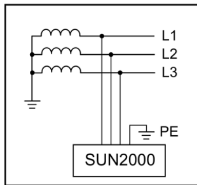
Figura 2-4 Sistema de alimentación de CA con puesta a tierra de punto neutral
