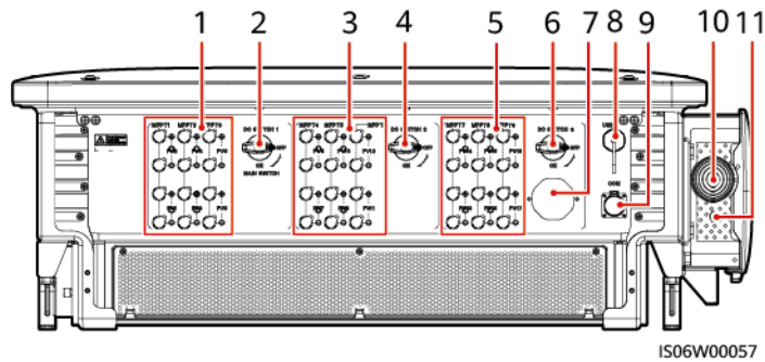
Figura 2-5 Ilustración de puertos (interruptor de CC manual)
