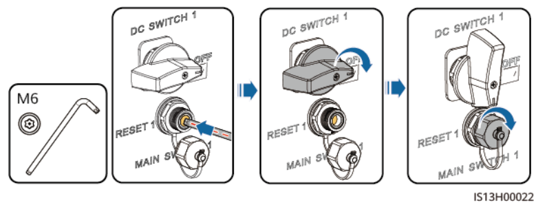
Figura 8-17 Restablecimiento y encendido del interruptor de CC (Se toma como ejemplo el DC SWITCH 1)
