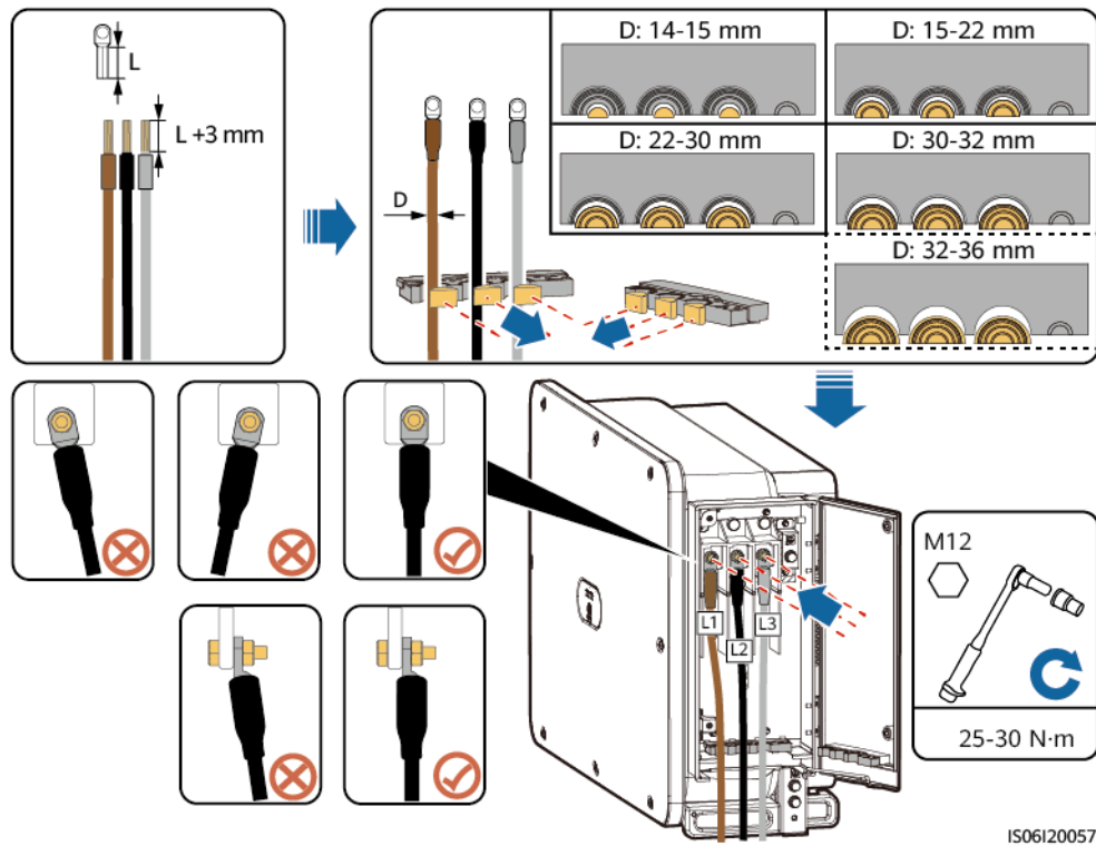
Figura 5-12 Conexión de cables
