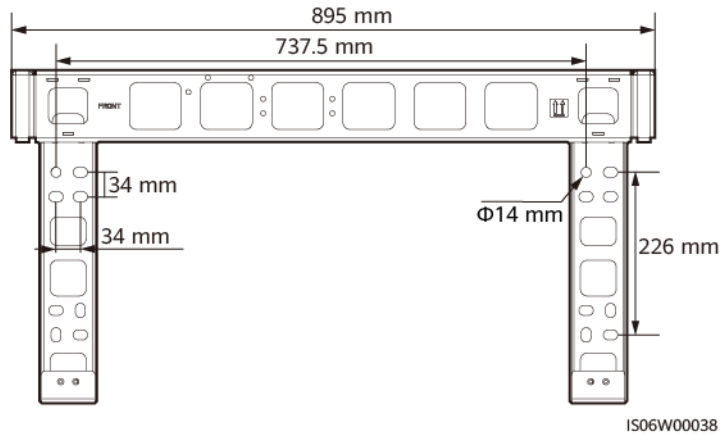
Figura 4-7 Dimensiones de la estructura de montaje
