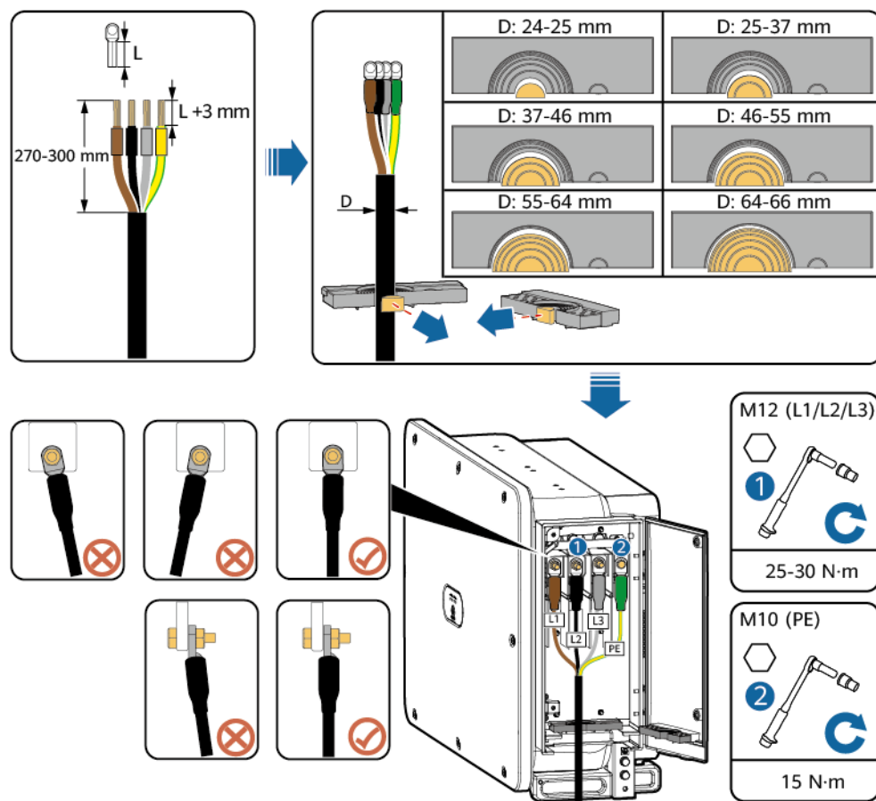
Figura 5-11 Conexión de cables
