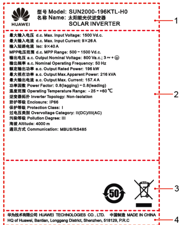
Figura 2-7 Placa de identificación (el SUN2000-196KTL-H0 se utiliza a modo de ejemplo)
