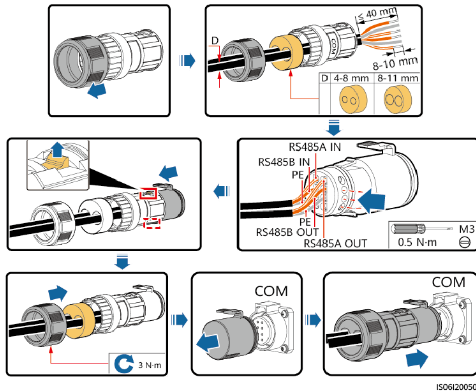
Figura 5-21 Conexión de cables (boquilla de goma de dos orificios de 4 a 8 mm)
