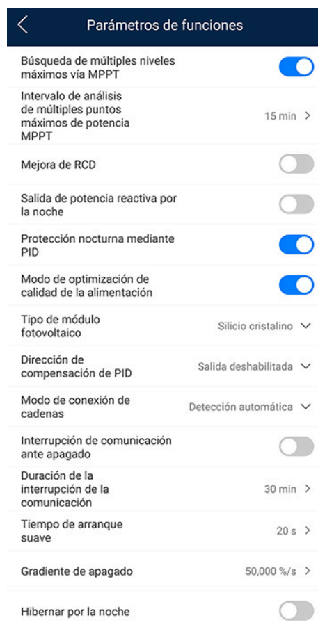
Figura 7-9 Parámetros de funciones (usuario avanzado)
