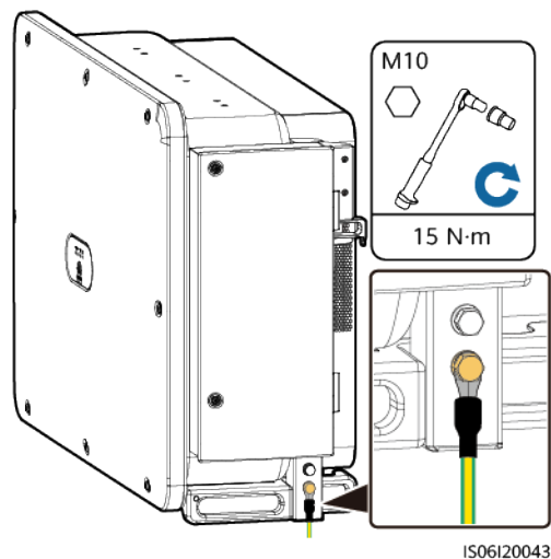
Figura 5-10 Conexión de cables
