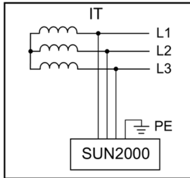
Figura 2-3 Red eléctrica admitida
