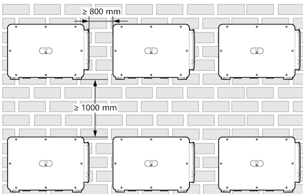
Figura 4-6 Modo de instalación apilado (no recomendado)
