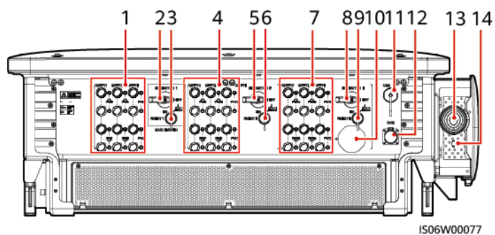
Figura 2-6 Ilustración de puertos (interruptor de CC automático)
