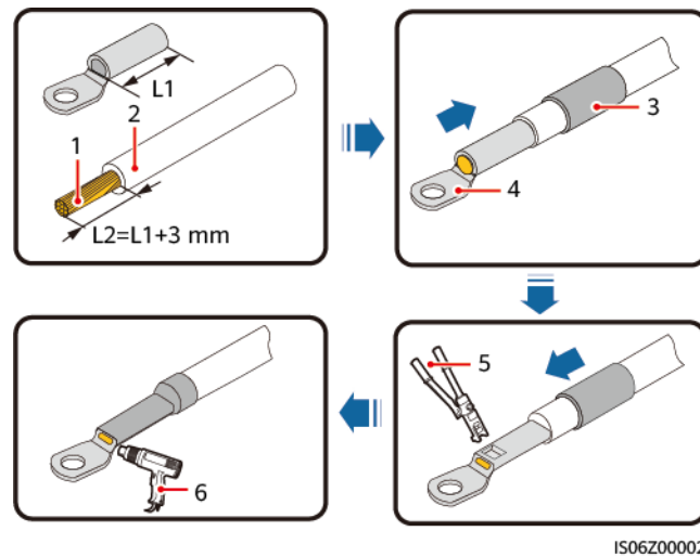
Figura 5-3 Crimpado del terminal DT
