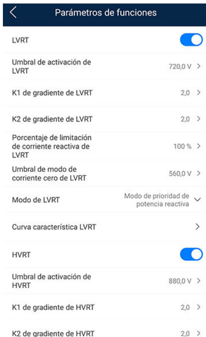
Figura 7-12 Parámetros de funciones (usuario especial)
