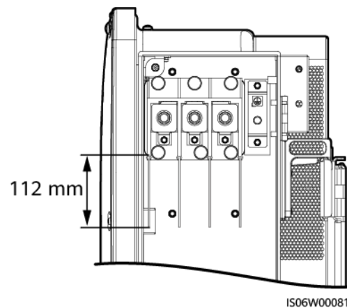
Figura 5-9 Especificación de la placa deflectora
