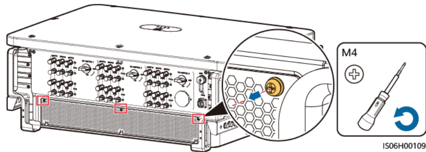
Figura 8-2 Retiro del amortiguador
