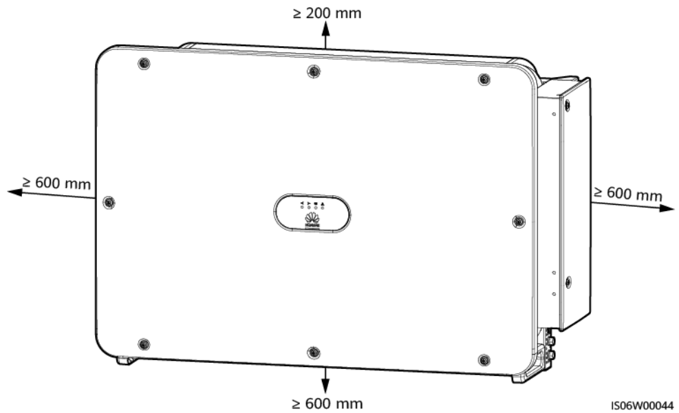
Figura 4-2 Espacio de instalación
