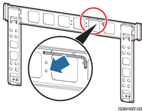
Figura 4-8 Extracción de la llave torx de seguridad
