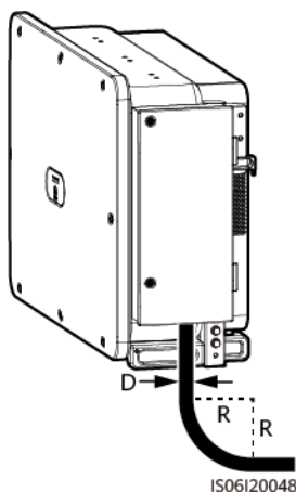
Figura 5-13 Radio de curvatura
