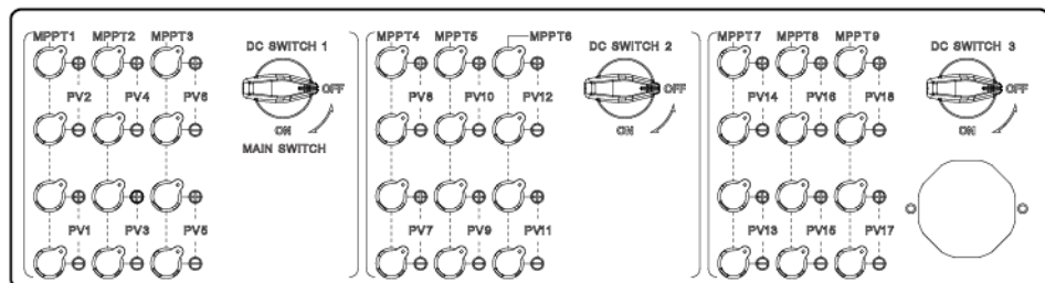
Figura 5-14 Bornes de CC
