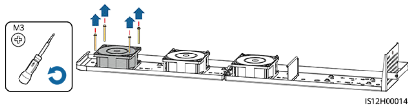
Figura 8-9 Desmontaje del ventilador
