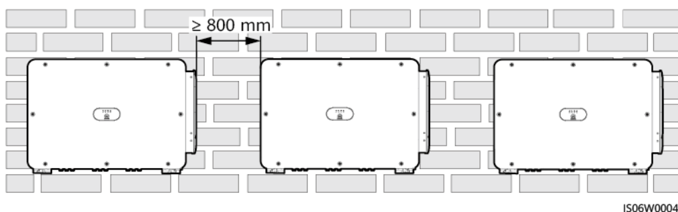
Figura 4-4 Modo de instalación horizontal (recomendado)
