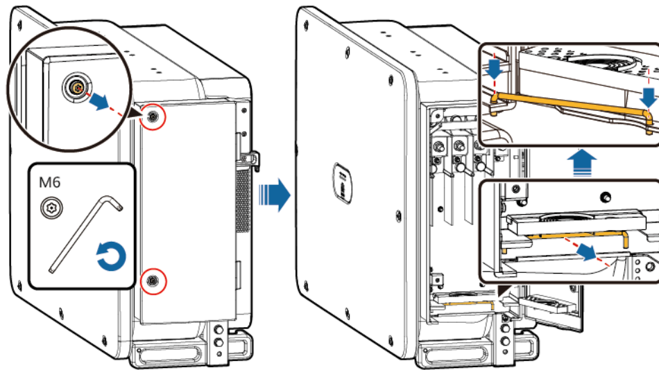
Figura 5-4 Apertura de la puerta del compartimento de mantenimiento
