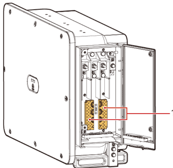
Figura 5-5 Cómo extraer accesorios del compartimento de mantenimiento
