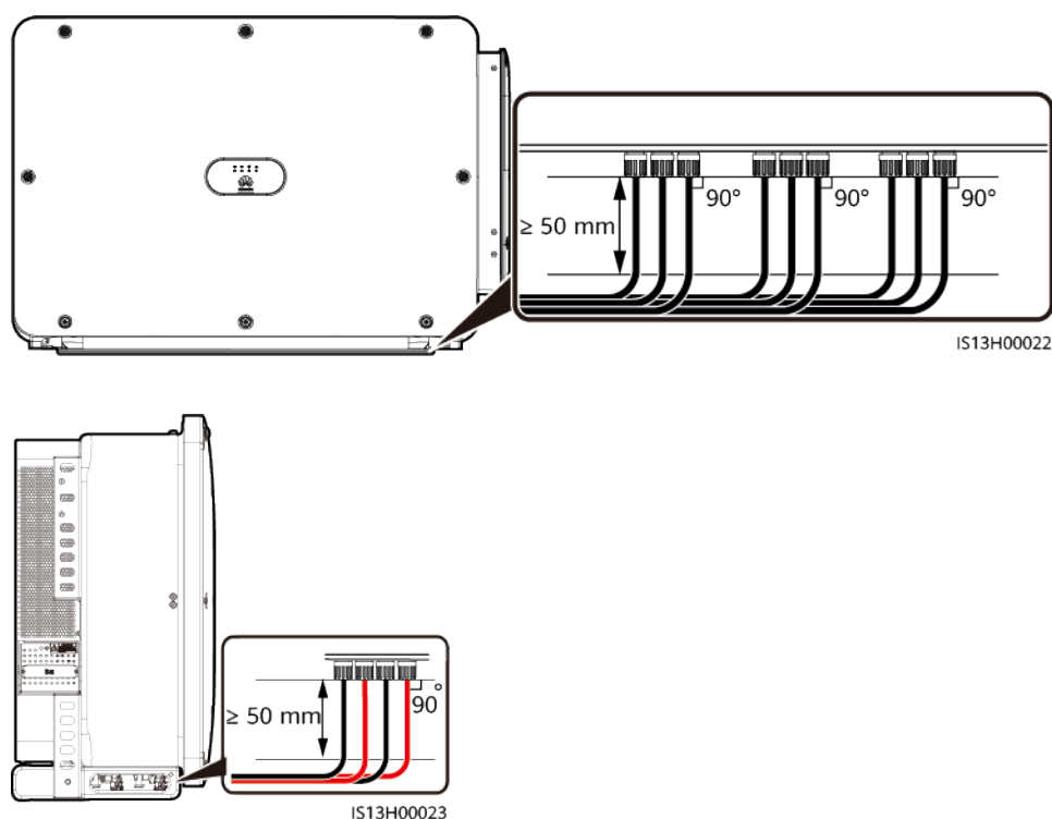
Figura 5-18 Requisitos del proceso de cableado de alimentación de entrada de CC
